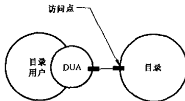
图 1 访问目录
