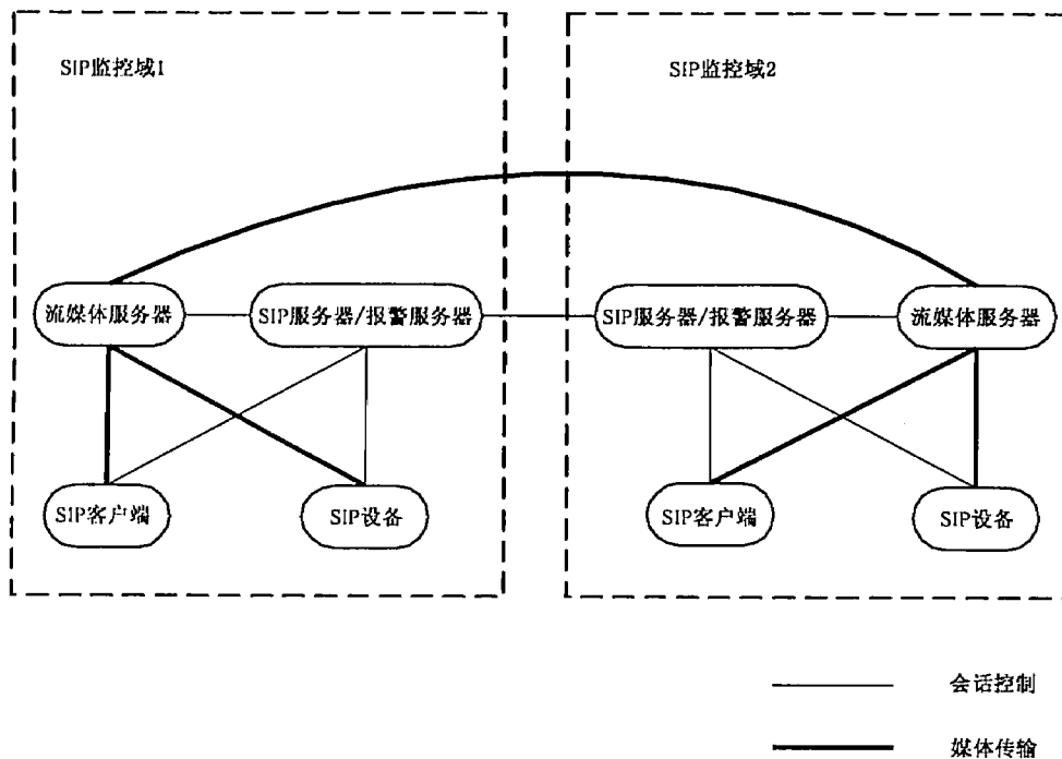
图 1 SIP 监控域互联结构示意图
